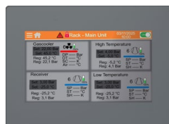
Ecrã ET6 de 7"
